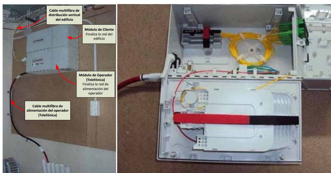
Ilustración 17-1. Caja terminal óptica (CTO) interior.
