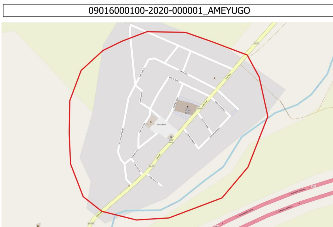
Ilustración 13. Área de despliegue FTTH en sombreado gris.
