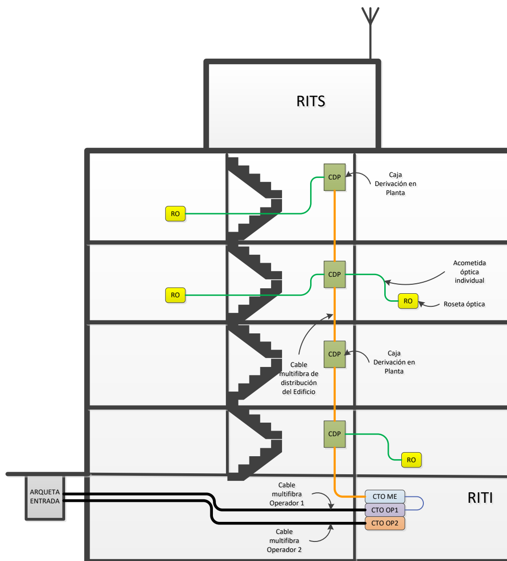
Ilustración 16. Vertical de edificio con despliegue por interior.
