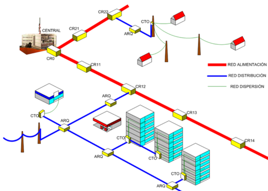
Ilustración 12. Arquitectura FTTH.
